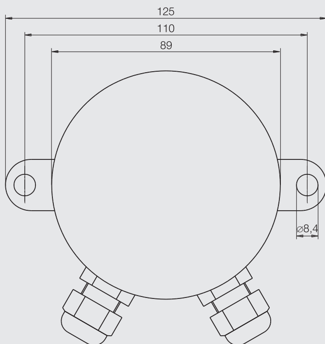
Размерный чертёж электронного блока
