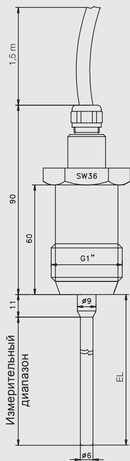
Размерный чертёж NSK-387.1
