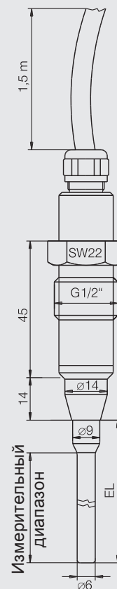
Размерный чертёж NSK-187
