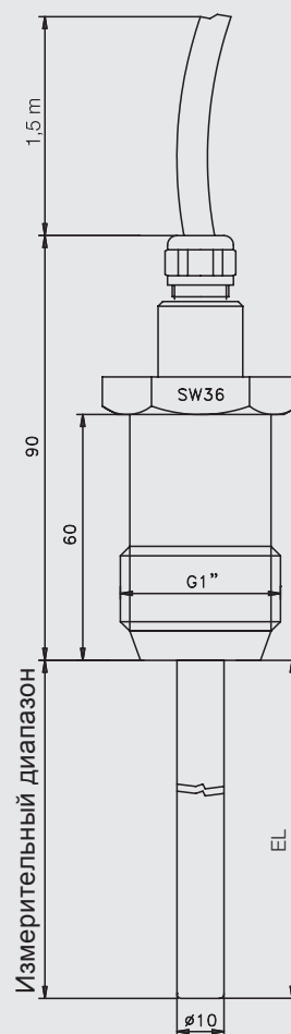
Размерный чертёж NSK-388 / ... / H
