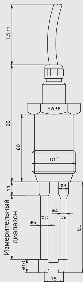
Размерный чертёж NSK-387.2
