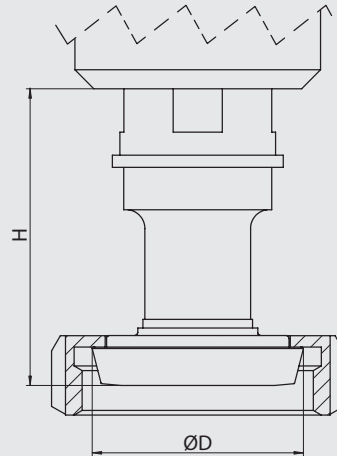
Taille DIN 11851
