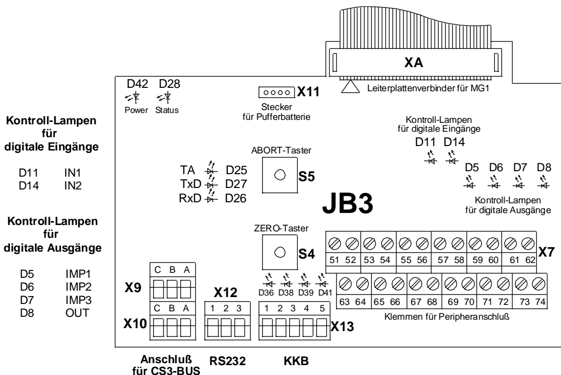
Abbildung: Junctionboard JB3
