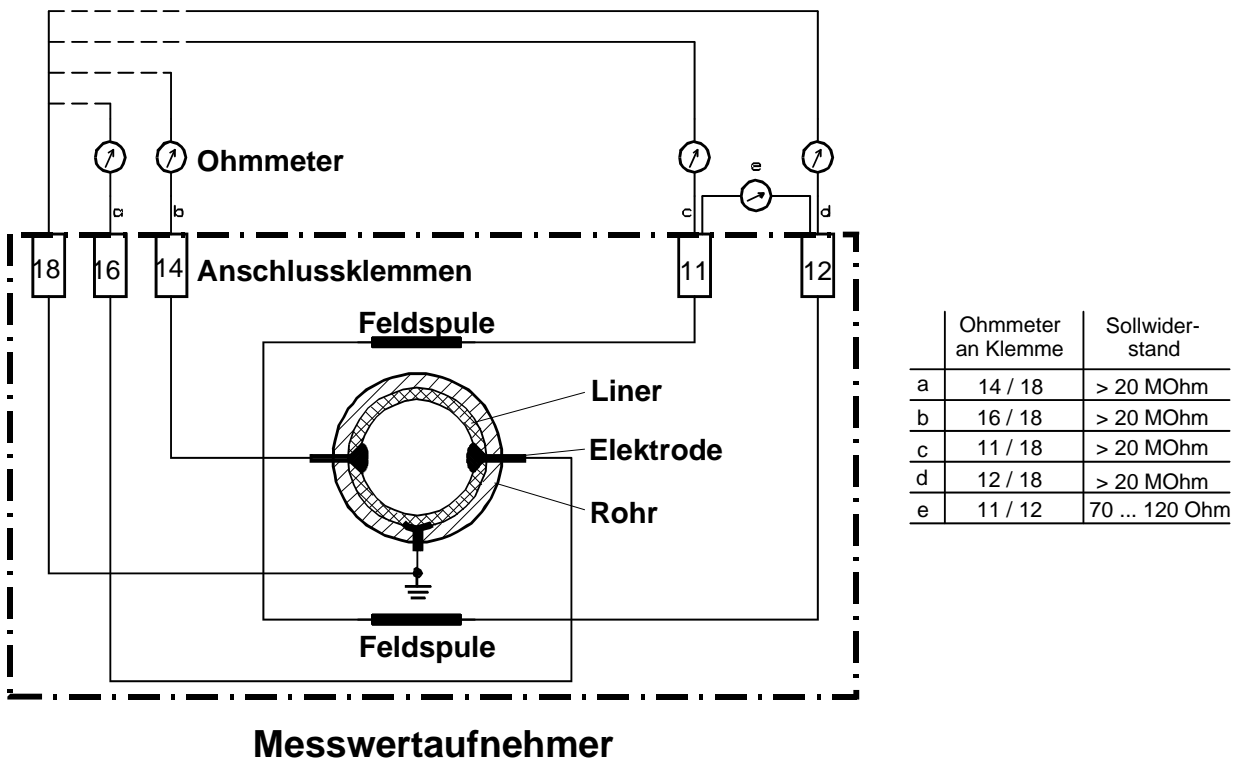
Abbildung: Isolationsprüfung
